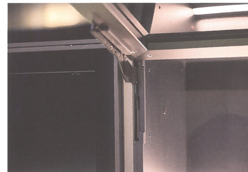
Het FREEslim flap-beslag kan op de zijwand worden gemonteerd, maar ook volledig worden ingefreesd.
